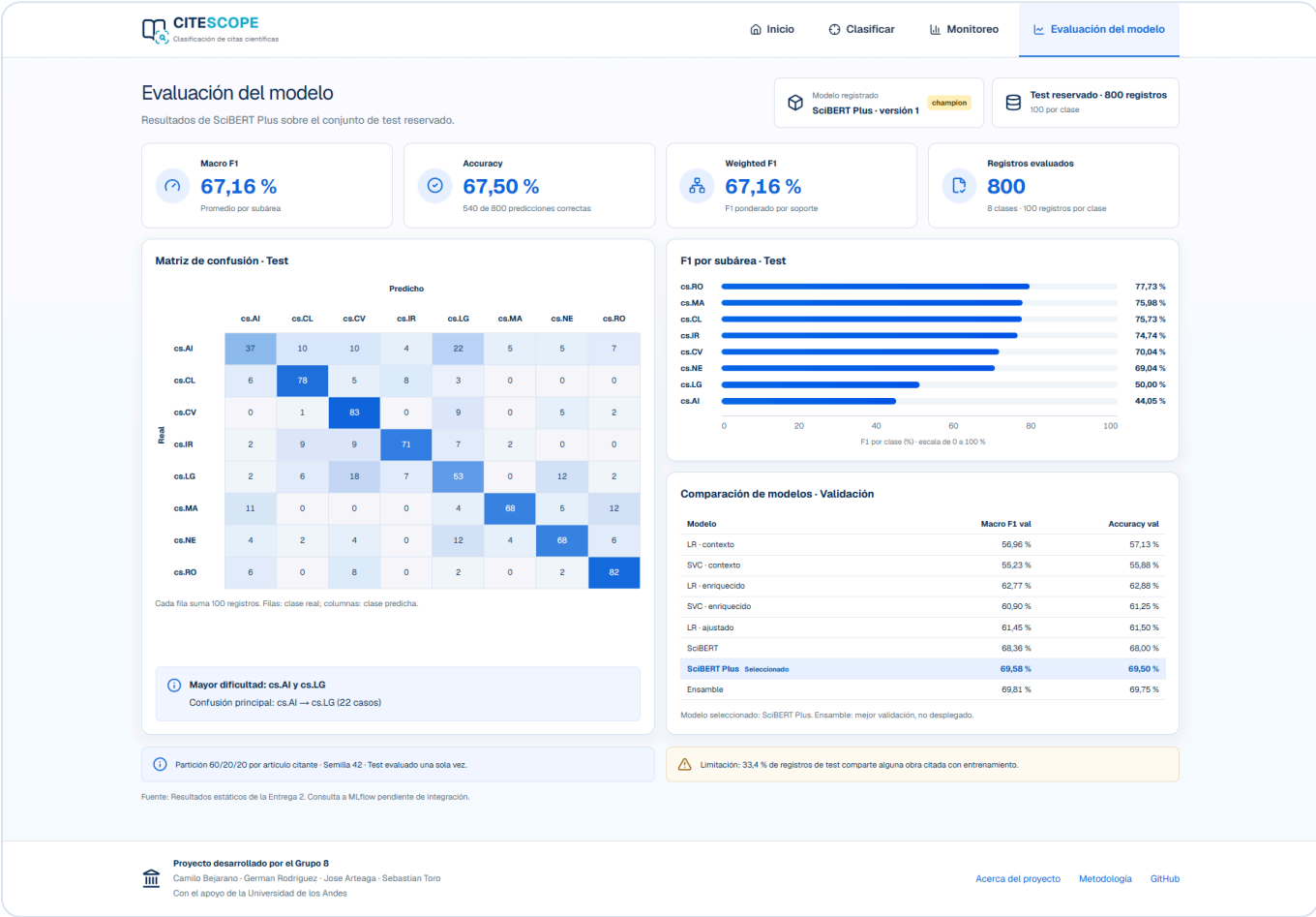
Figura 6. Evaluación de SciBERT Plus: métricas de test, matriz de confusión y comparación de validación.
